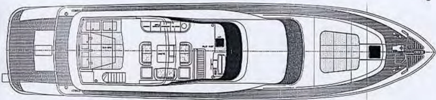
MAIORA 86' FLY-BRIDGE PLAN (SC. 1/50)
