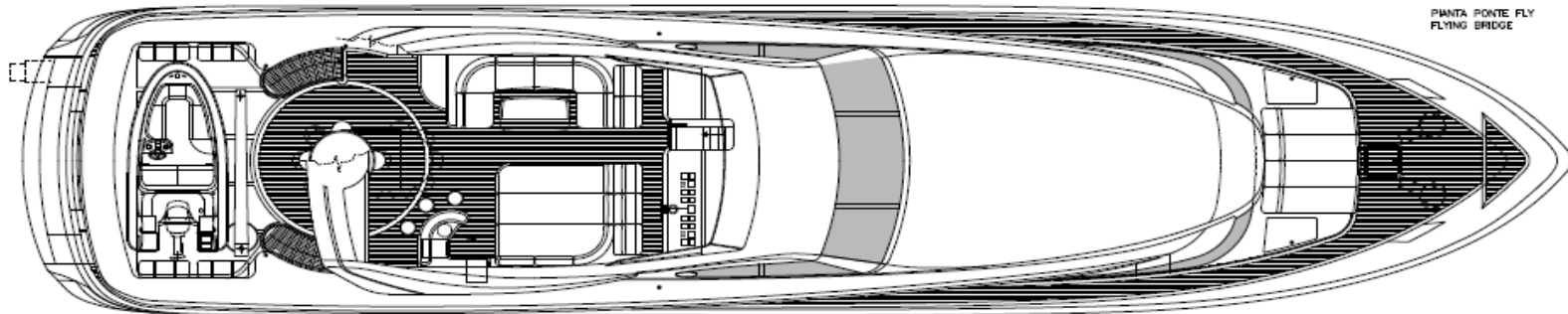
Pianta Ponte Coperta Main Deck
